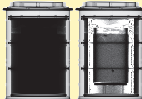
Links: Radiographie eines 280-L-Fasses mit eingestelltem 200-L-Fass und innerem Stahlbehälter mit zementiertem Abfall. Die Messdaten decken einen dynamischen Bereich von 16-Bit ab. Durch Anpassung der Graustufenskala können schwächer (links) bzw. stärker absorbierende Bereiche (rechts) visualisiert werden.
