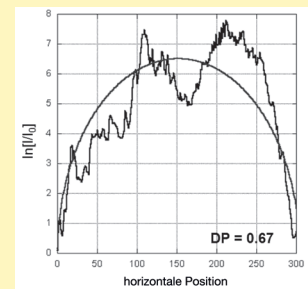
Linienprofil durch eine Höhenposition. Die glatte Kurve visualisiert die beste Anpassung an eine homogene Dichteverteilung
