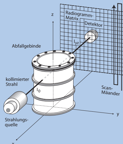
Prinzip der Digitalen Radiographie
